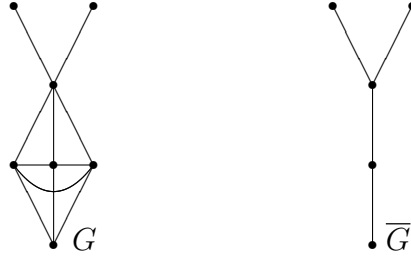
Рис. 2: Граф G и его сжатие \bar{G}
